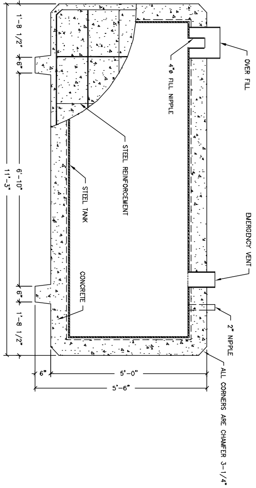
SECTION A-A
