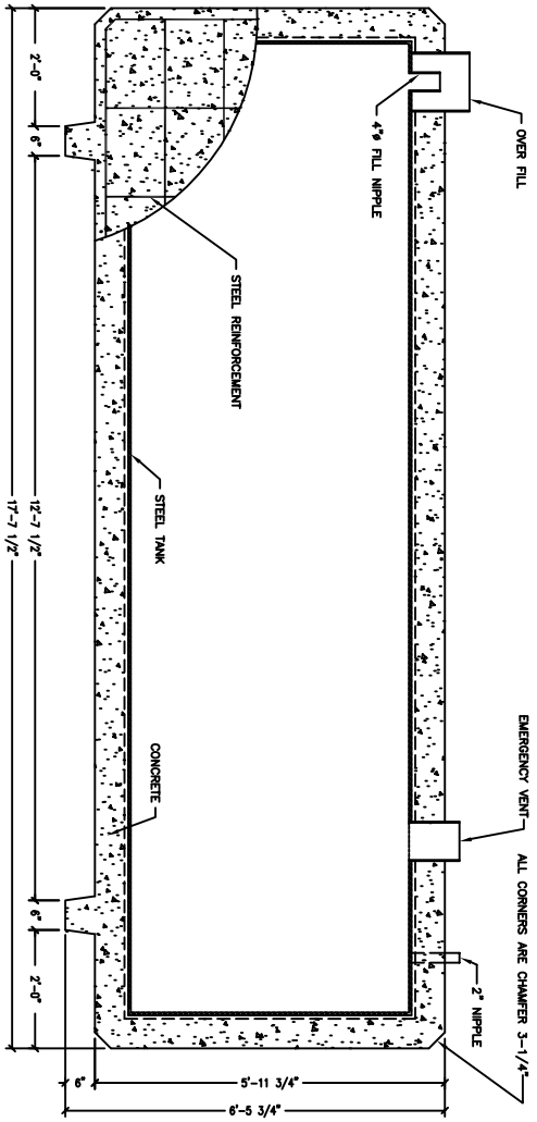
SECTION A-A
